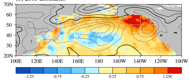
(b) 2005 anomalies
